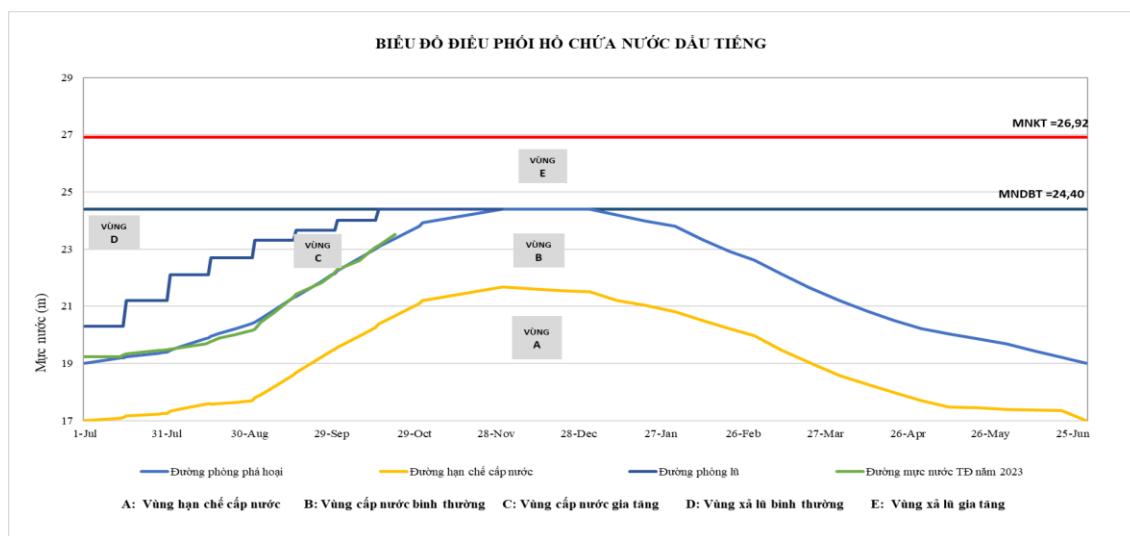
Hình 1: Biểu đồ điều phối hồ Dầu Tiếng
