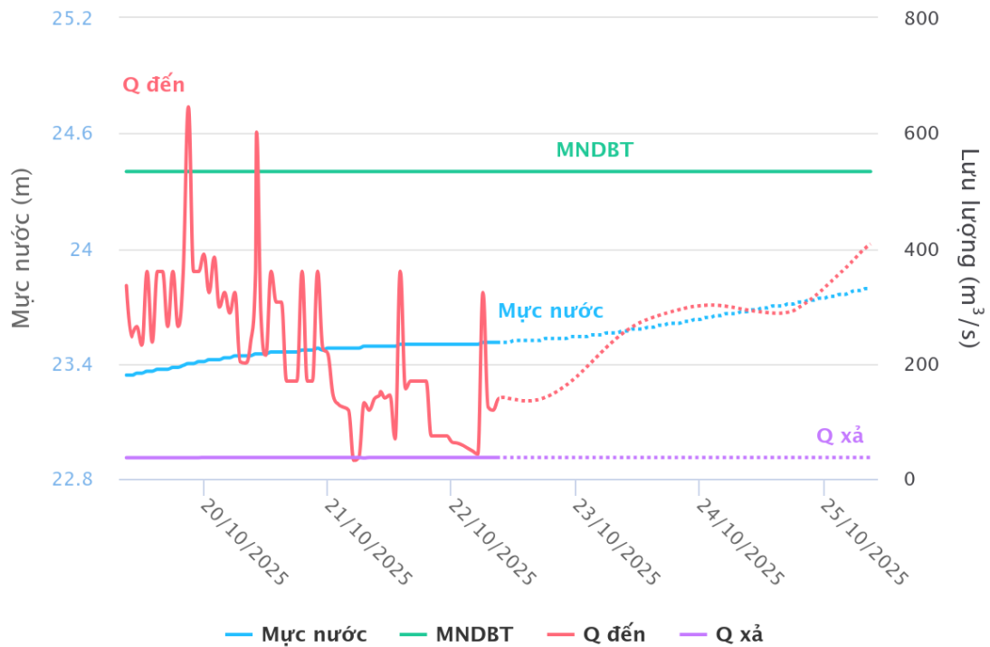
Hình 3: Phương án xả lũ hồ Dầu Tiếng
